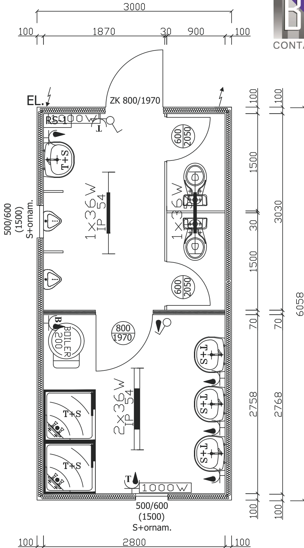
Standardsanitärcontainer Typ BC - 8 in 3 m Breite
