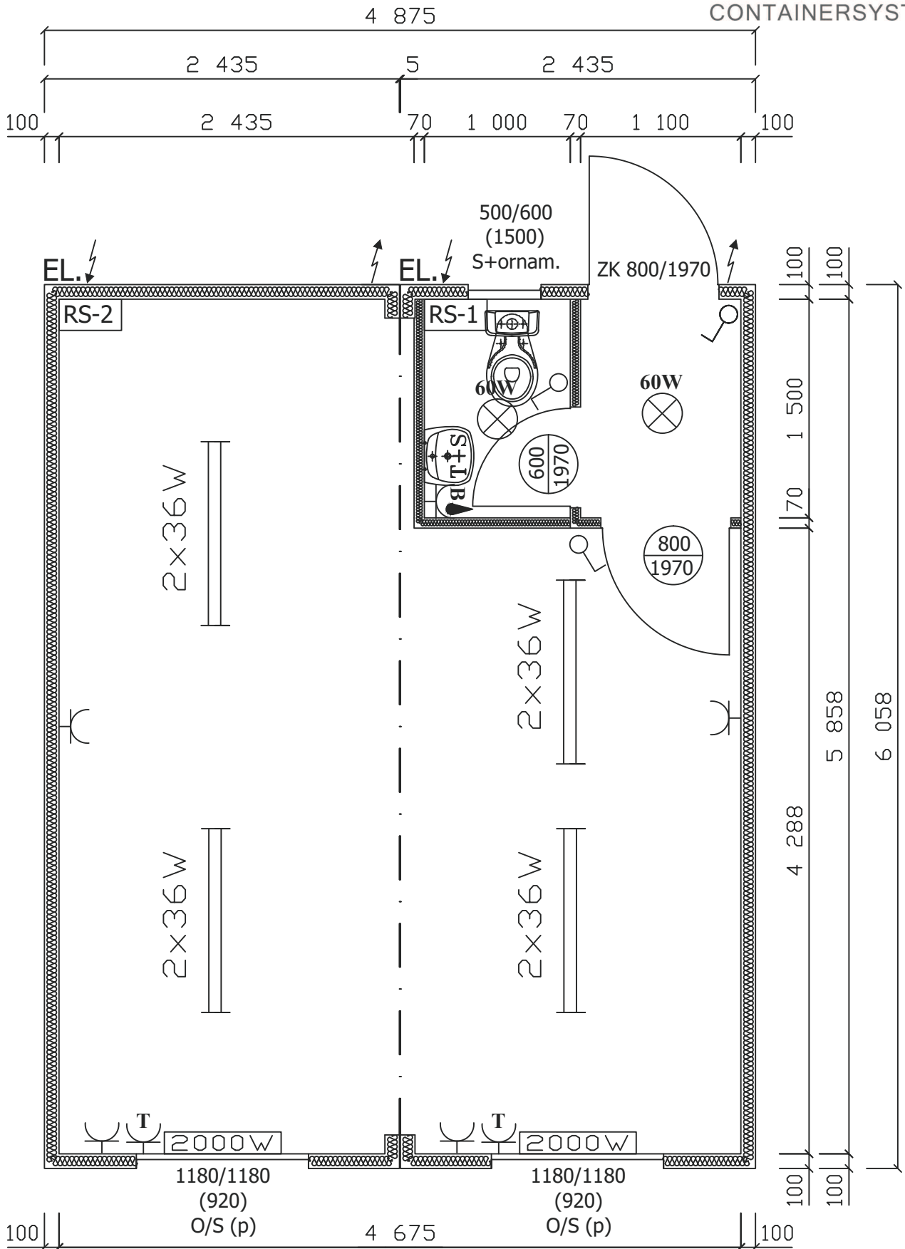
Standarddoppelcontainer Typ BC - 17
